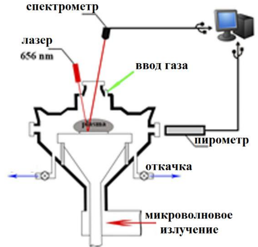
Схема реакционной камеры
